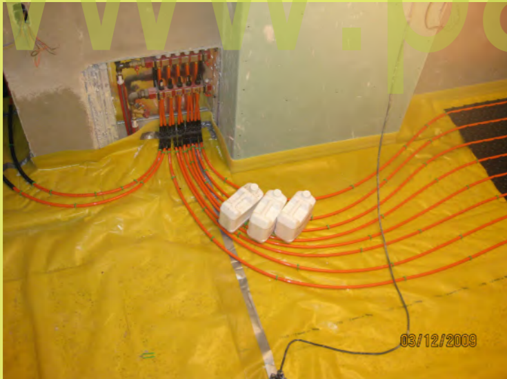
10_Der Verteiler im Erdgeschoss
