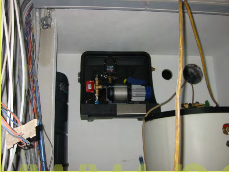
19_Und das ist das Regenwasserpumpwerk
