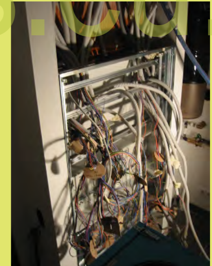
28_Viel Chaos im E-Verteiler
