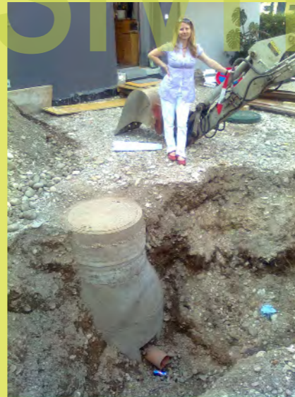
40_Am 25 Mai wird das Niveau des Kanalanschlusses berichtigt
